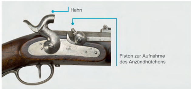
Abb. 15: Perkussionsschloss offen
