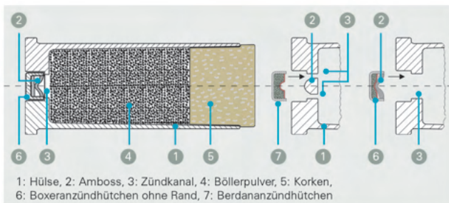
Abb. 16: Schnitt durch eine geladene Kartusche mit Boxeranzündung (links), Kartusche mit Berdananzündung (Mitte), Kartusche mit Boxeranzündung (rechts)
